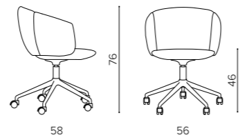
NT 409C MINI 5-spoke aluminum swivel base on casters base girevole a 5 razze in alluminio su ruote piétement pivotant en aluminium à 5 branches sur roulettes
