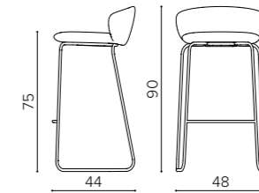
NT75U05 STOOL stackable stool with steel sled base sgabello impilabile con base a slitta in acciaio tabouret empilable avec piétement luge en acier
