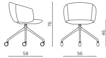
NT 4096R MINI 4-spoke polypropylene swivel base on casters base girevole in polipropilene a 4 razze su ruote piétement pivotant à 4 branches en polypropylène sur roulettes
