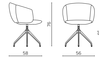
NT 4098 MINI 4-spoke aluminum swivel base base girevole in alluminio a 4 razze piétement pivotant en aluminium à 4 branches
