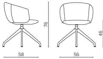
NT 4096 MINI 4-spoke swivel polypropylene base base girevole in polipropilene a 4 razze piétement pivotant à 4 branches en polypropylène
