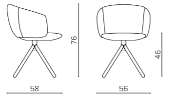
NT 4090 MINI 4-spoke steel base base girevole a 4 razze in acciaio piétement pivotant à 4 branches en acier
