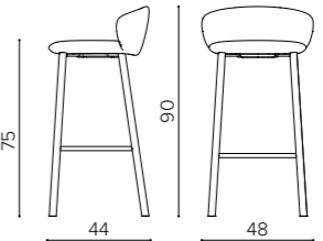
NT75U09 STOOL stool with 4 wooden legs sgabello con 4 gambe in legno tabouret avec 4 pieds en bois
