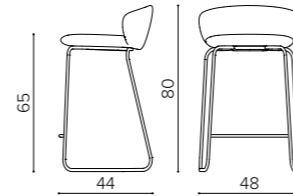
NT65U05 STOOL stackable stool with steel sled base sgabello impilabile con base a slitta in acciaio tabouret empilable avec piétement luge en acier
