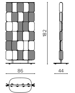
PA 0818 MIX acoustic panel pannello acustico séparateur acoustique
