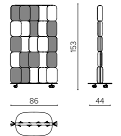
PA 0815R MIX acoustic panel with castors pannello acustico con ruote séparateur acoustique avec roues
